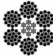
6 x 25 FW (Filler Wire)
