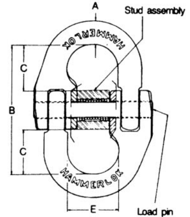
CM Hammerlok Coupling Link
