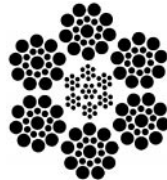
6 x 19 Seale (7 x 7 IWRC)
