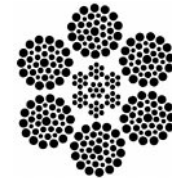
6 x 36 WS (Warrington Seale)
