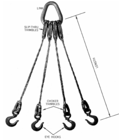
6 Part/U-8
