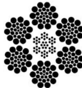
6 x 26 WS (Warrington Seale)
