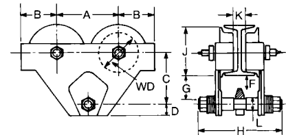
1/4, 1/2, 1 and 2 Ton
