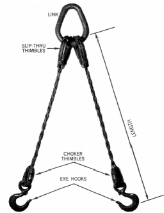
8 Part/U-6
