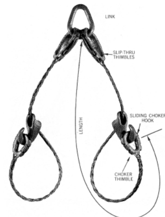
6 Part/U-4
