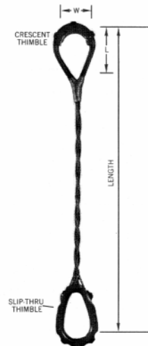
8 Part/U-1
