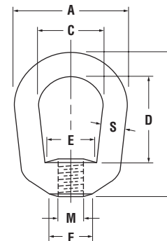
G-400 Eye Nuts
