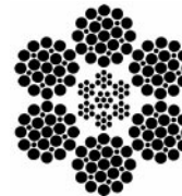
6 x 25 Filler Wire (7 x 7 IWRC)
