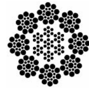
8 x 19 Seale (IWRC)
