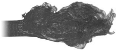
Tensile Break
