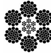
6 x 31 WS (Warrington Seale)
