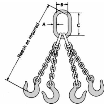
QOS Sling Hooks
