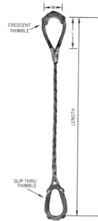
6 Part/U-1
