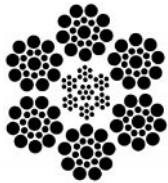
6 x 19 S (Seale)
