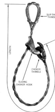
8 Part/U-3
